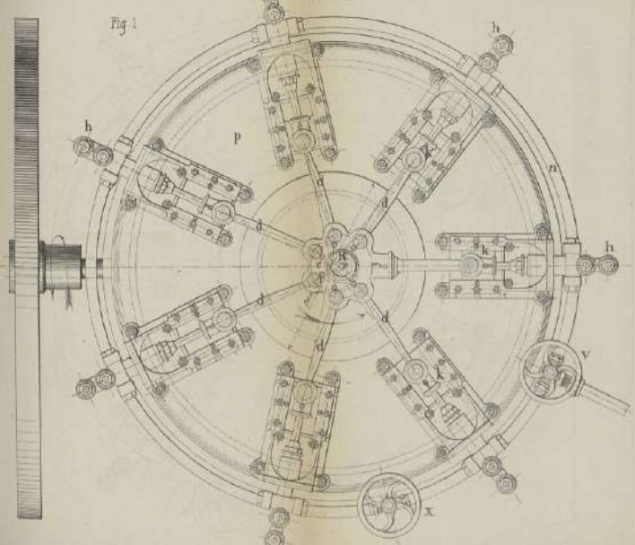
Ensemble de la pompe Echelle de 1/2"
