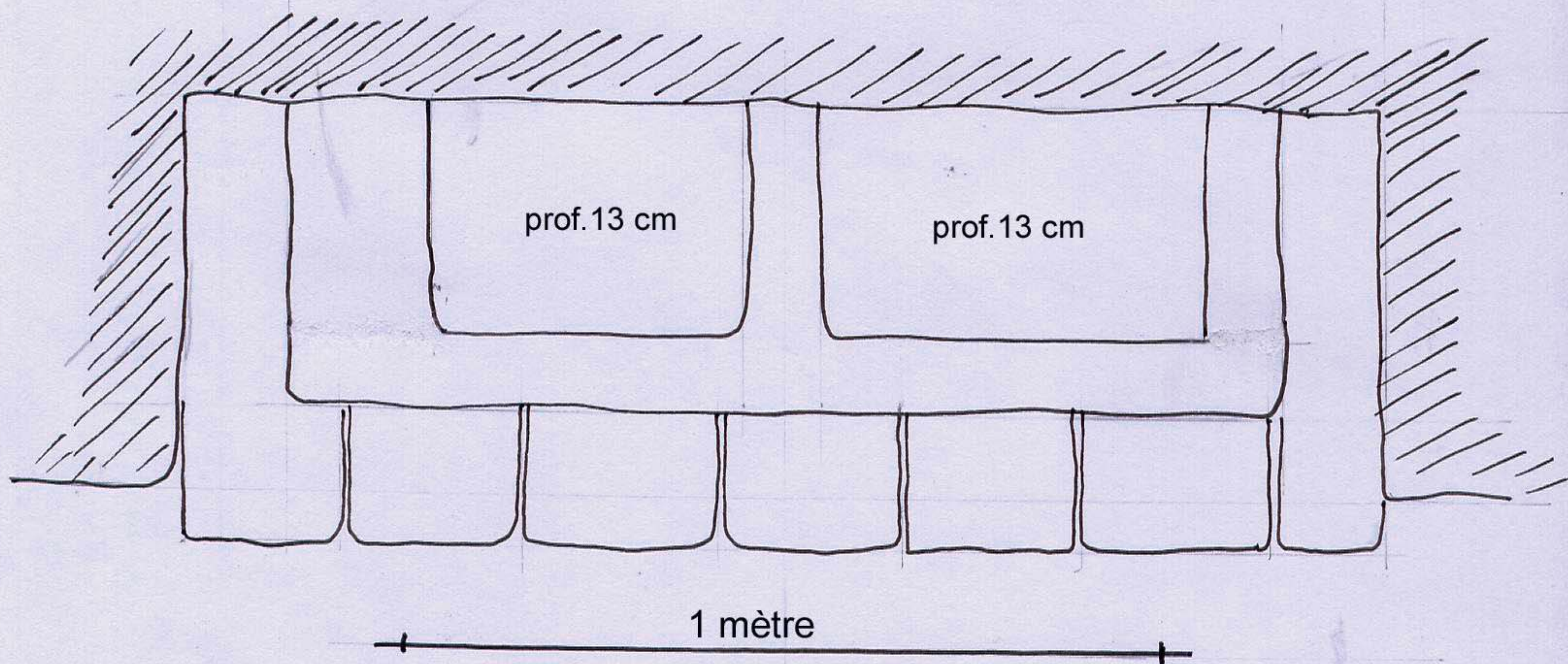
ELEVATION
