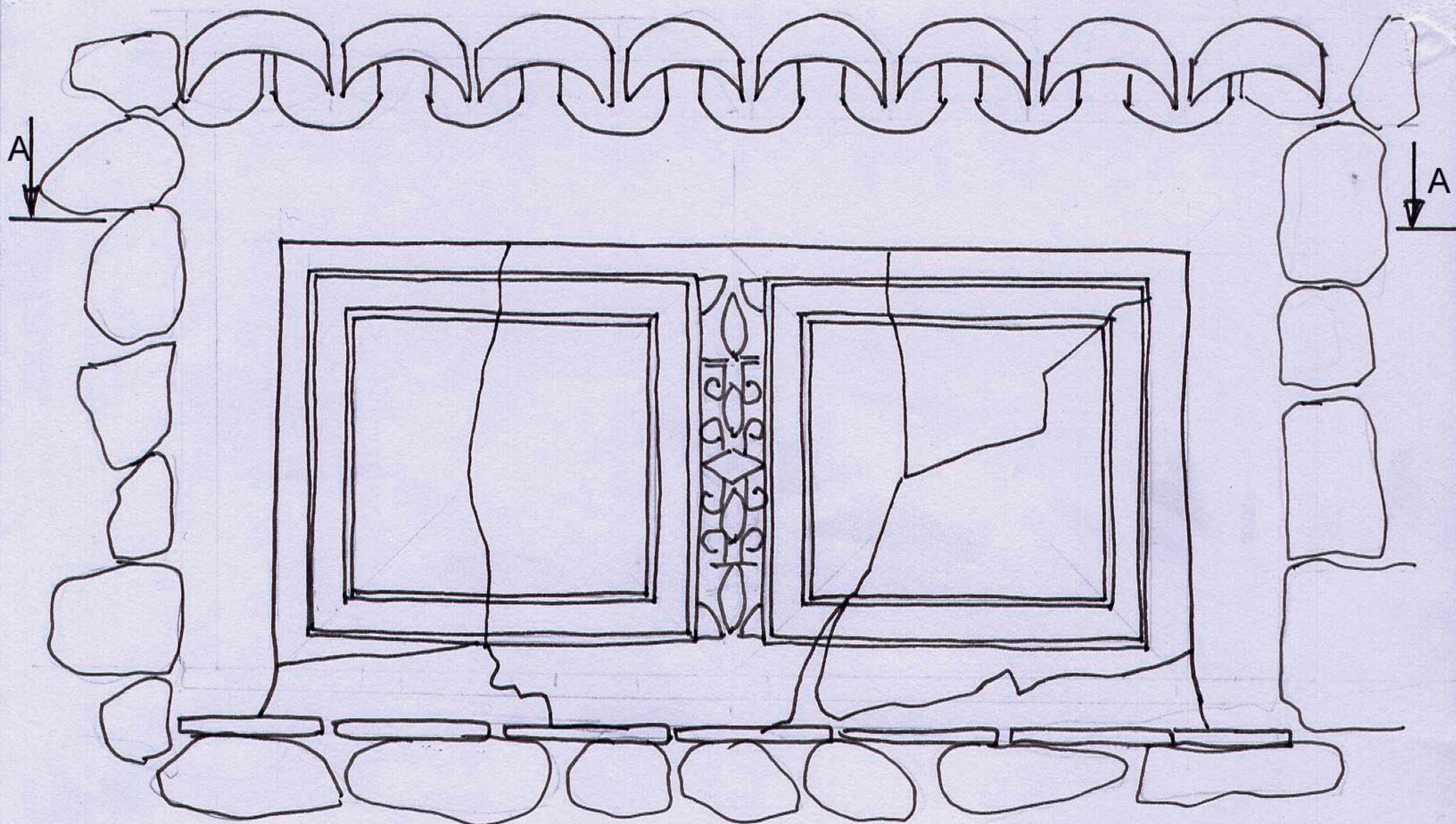
ELEVATION
