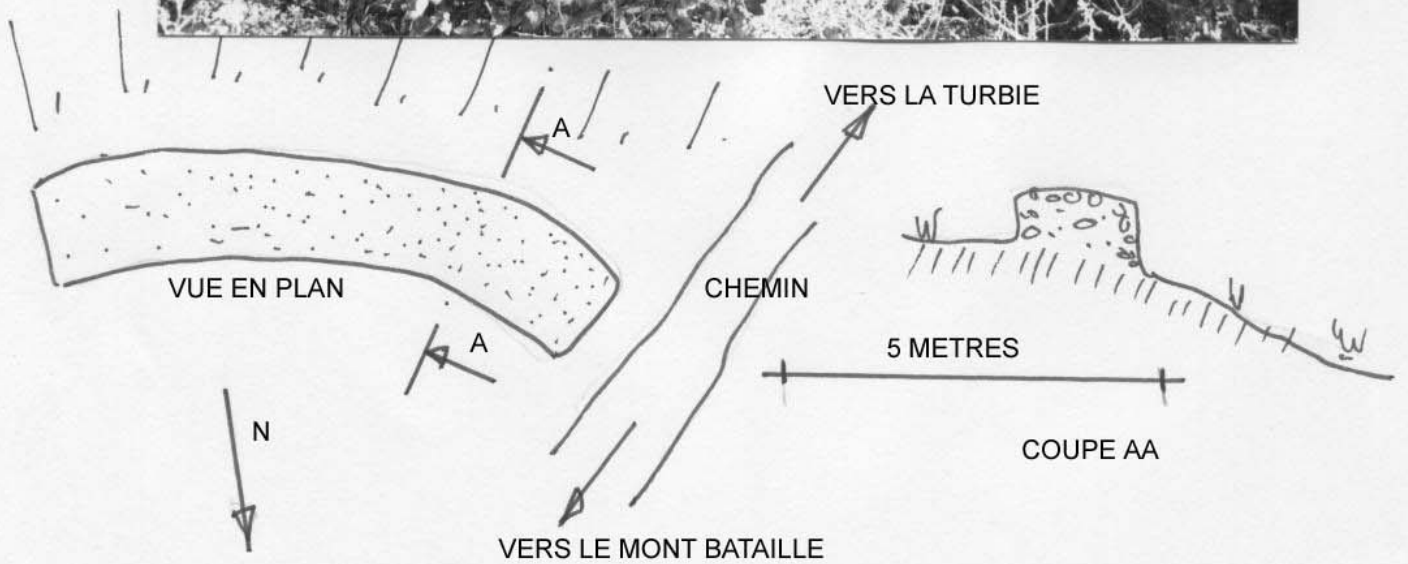
OUVRAGE AVANCE P1 - SUD DU MONT BATAILLE photo du haut: vu de l'amont - photo du bas: vu de l'aval
